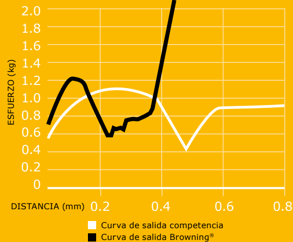
Curva típica, desplazamiento cola del disparador- esfuerzo en cola del disparador
